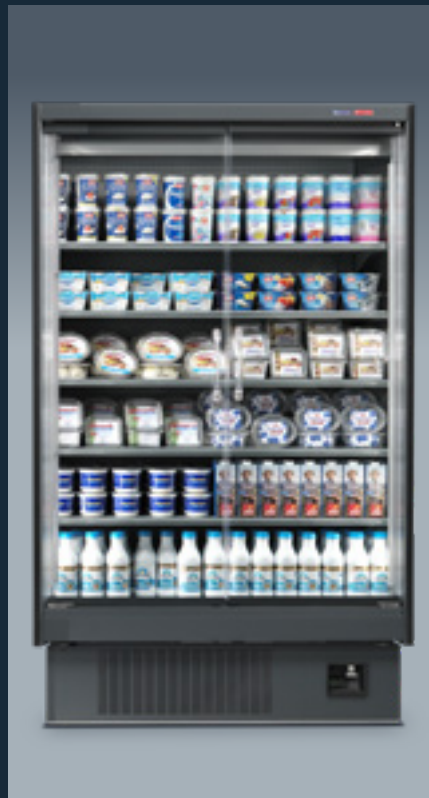
Porte "full vision" (optional). Full vision doors (optional). Vollsicht-Türen (optional). Portes panoramiques "full vision" (en option). Puertas "full vision" (opcionales). Полнообзорные двери (по заказу).
