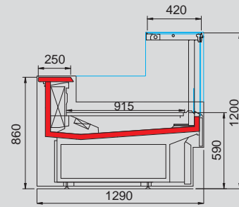
VDA2 Ventilato - Ventilated
